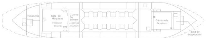
Vista bajo cubierta principal
